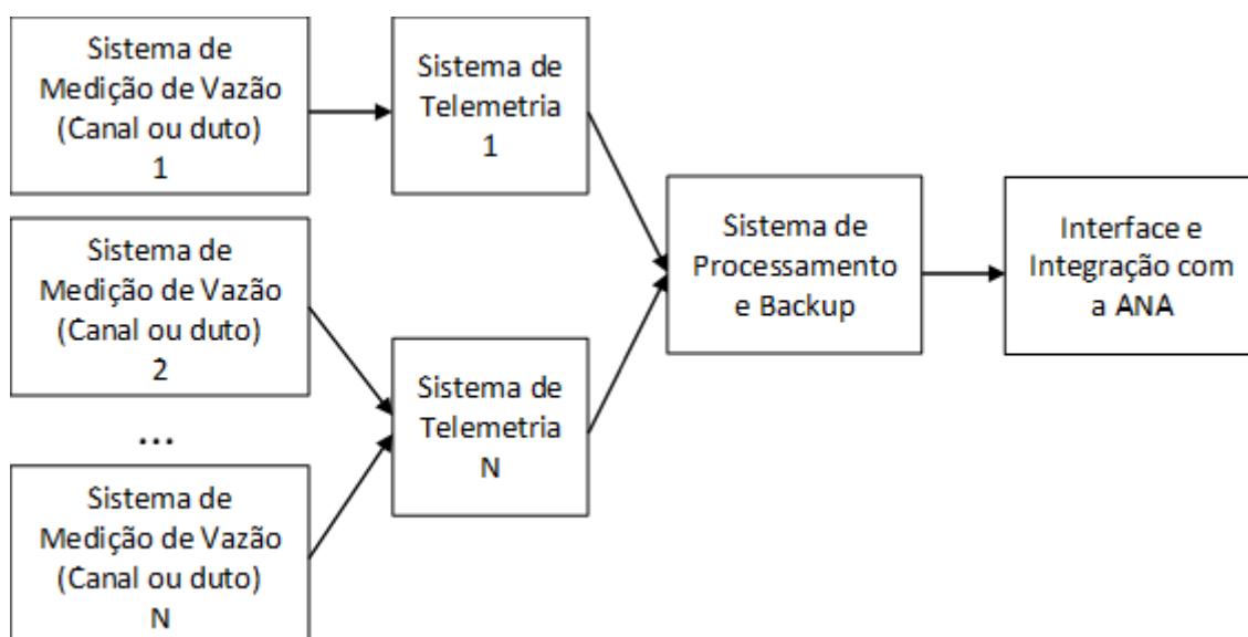
Figura 2 - Esquemático básico de integração entre os sistemas a serem executados pela contratada, conforme necessidade de adequação ao leiaute das instalações locais.
