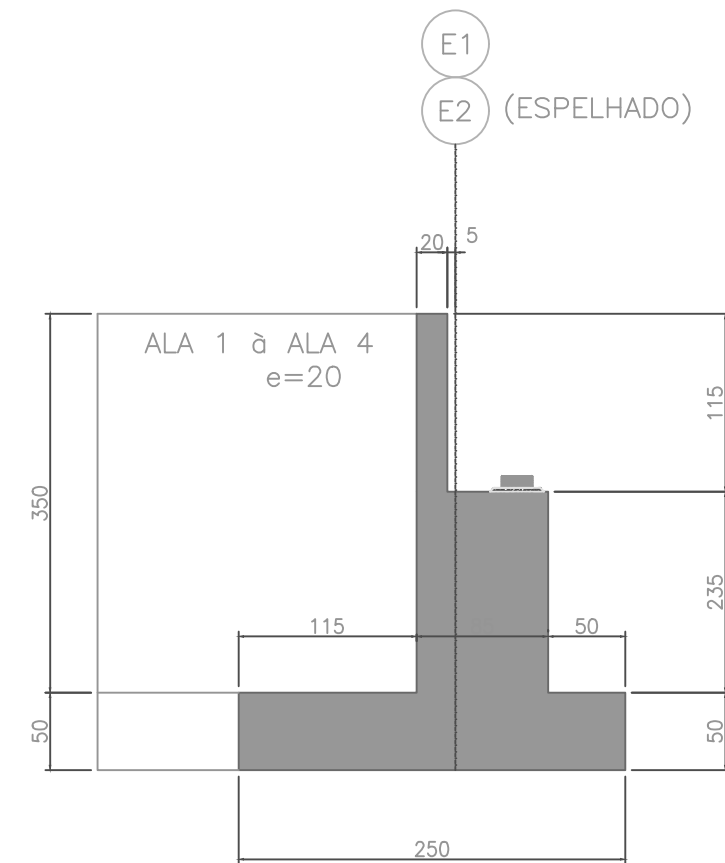
ENCONTROS E1/E2 ESC. SEM ESCALA
