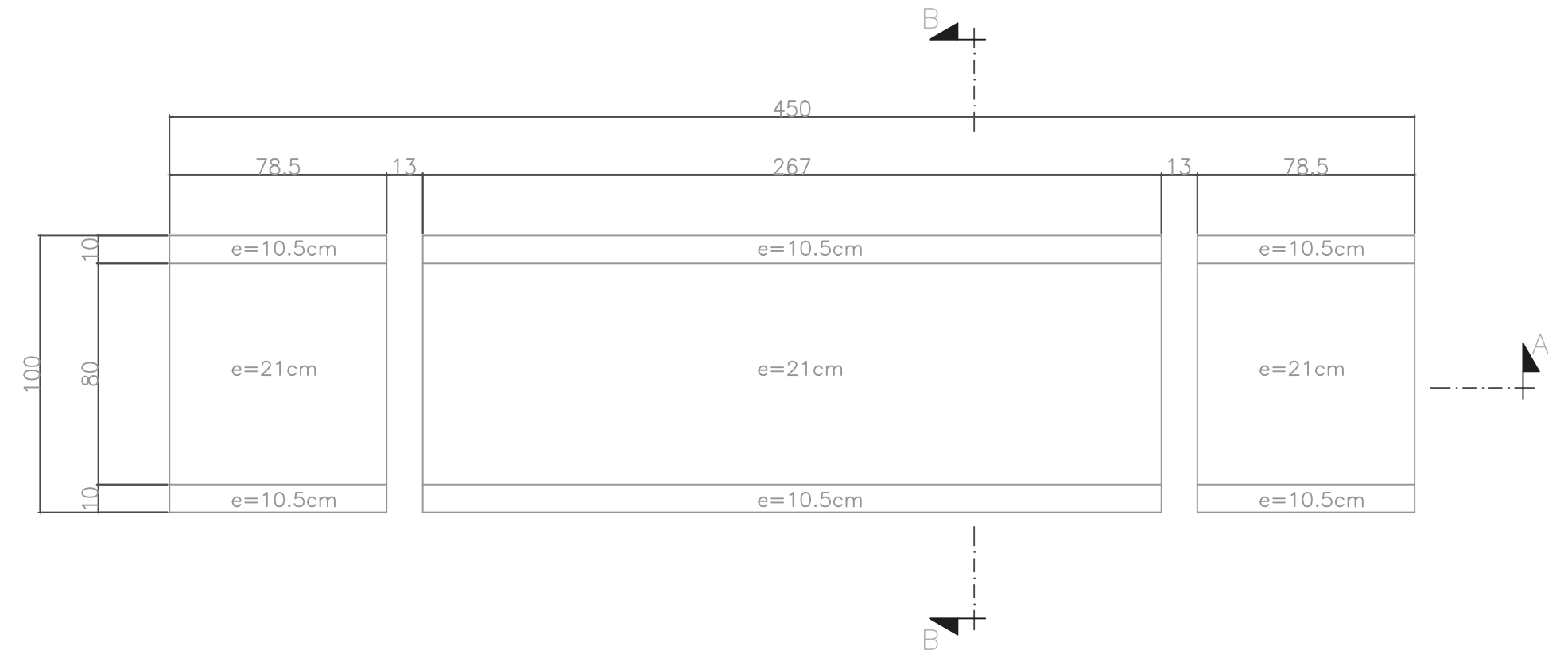
PLANTA DAS LAJES PRÉ-MOLDADAS ESC. SEM ESCALA
