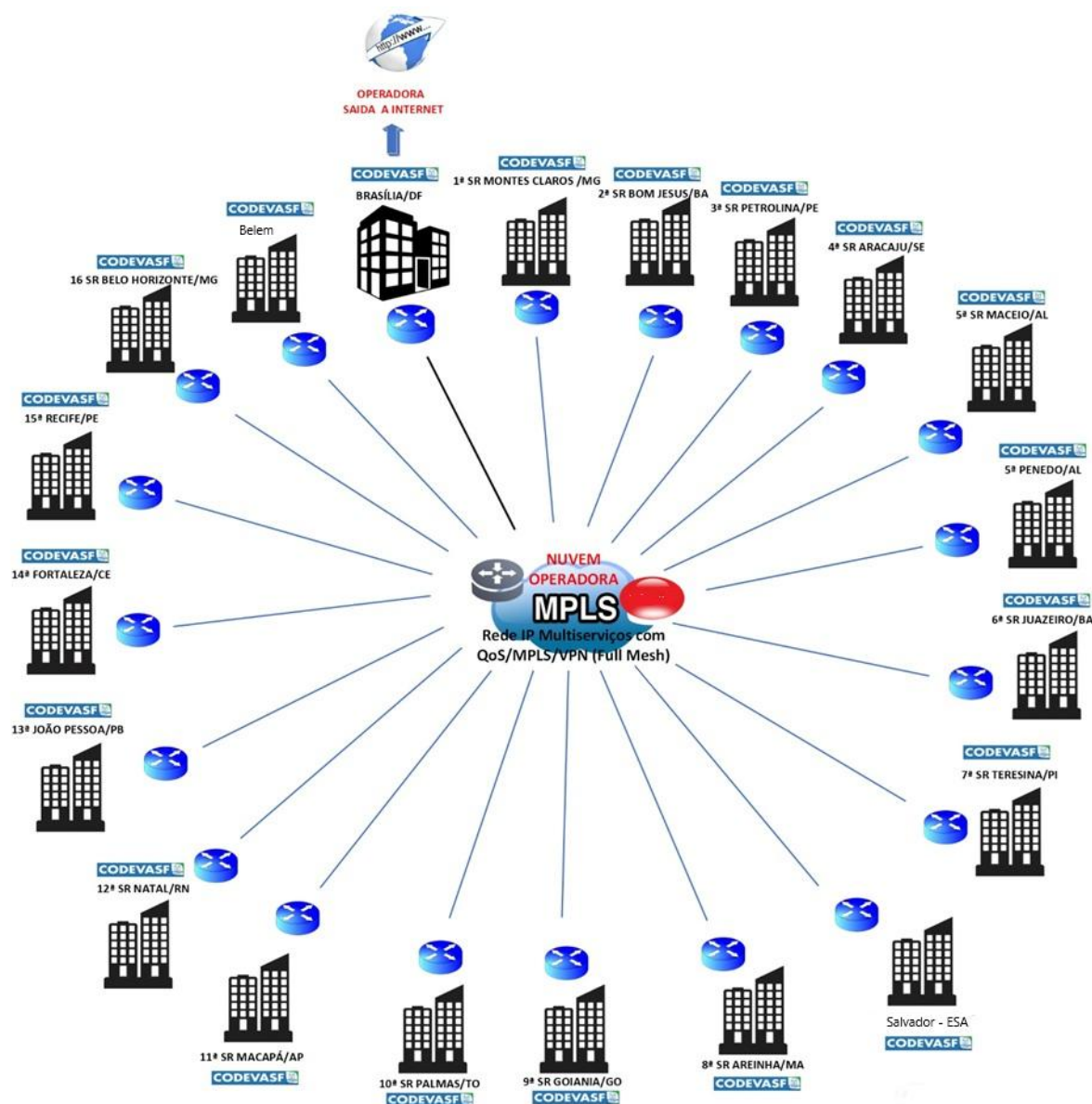
Figura 1 - Topologia da Rede WAN CODEVASF
