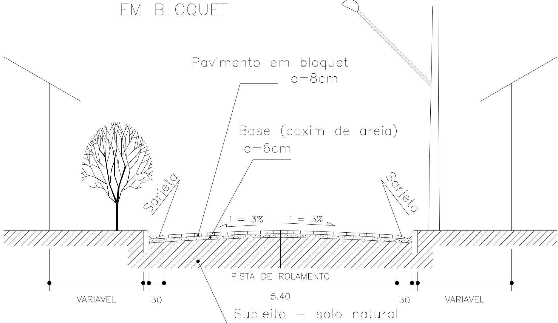
CORTE ESQUEMATICO DE PAVIMENTAÇÃO ESCALA: 1:6
