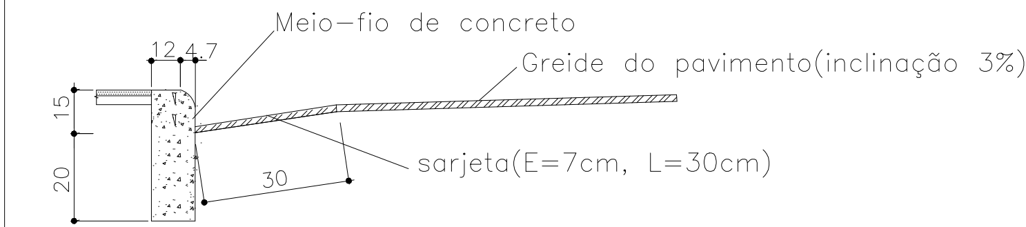
CORTE ESQUEMATICO DE GUIA E MEIO FIO ESCALA: 1:3
