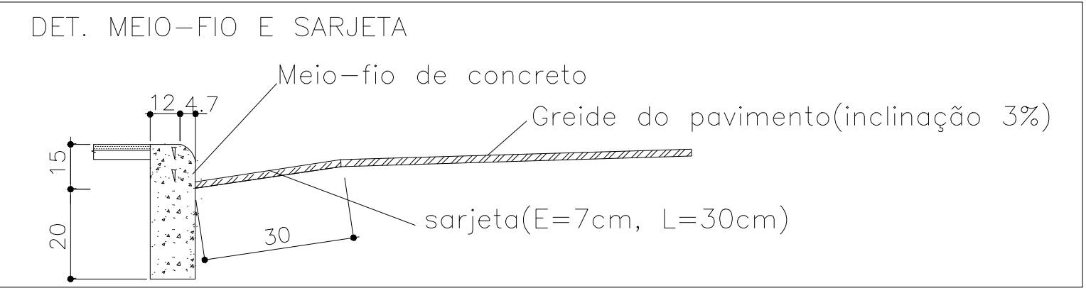
CORTE ESQUEMATICO DE GUIA E MEIO FIO ESCALA: 1:3
